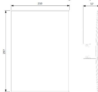
Afdekkap binnen bovenkant in voor- en zijaanzicht
