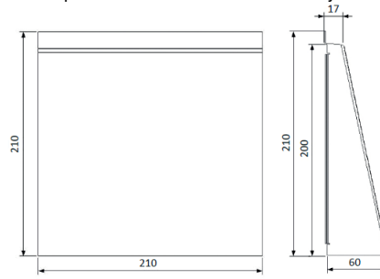
Afdekkap buiten bovenkant in voor- en zijaanzicht
