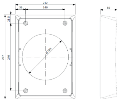
Afdekkap binnen onderkant in voor- en zijaanzicht
