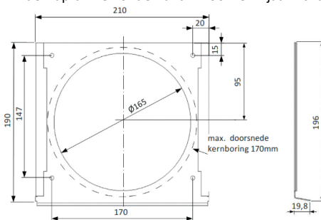
Afdekkap buiten onderkant in voor- en zijaanzicht
