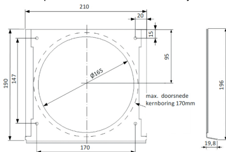
Afdekkap buiten onderkant in voor- en zijaanzicht
