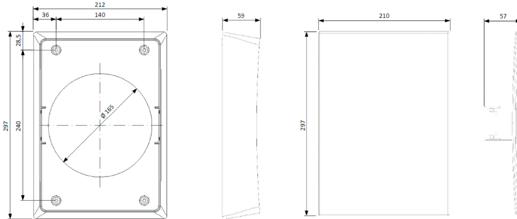
Afdekkap binnen onderkant in voor- en zijaanzicht
