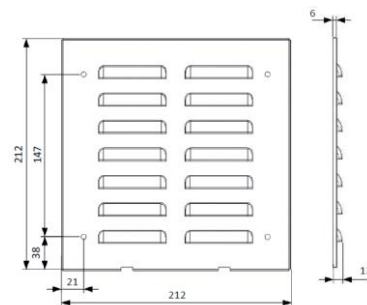
Beschermrooster Light in voor- en zijaanzicht
